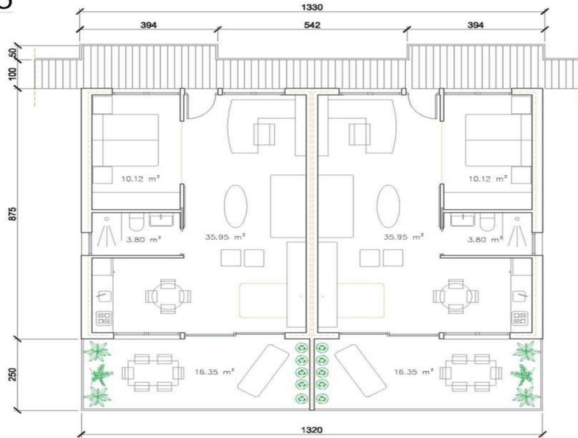
PLANTA ALTA
